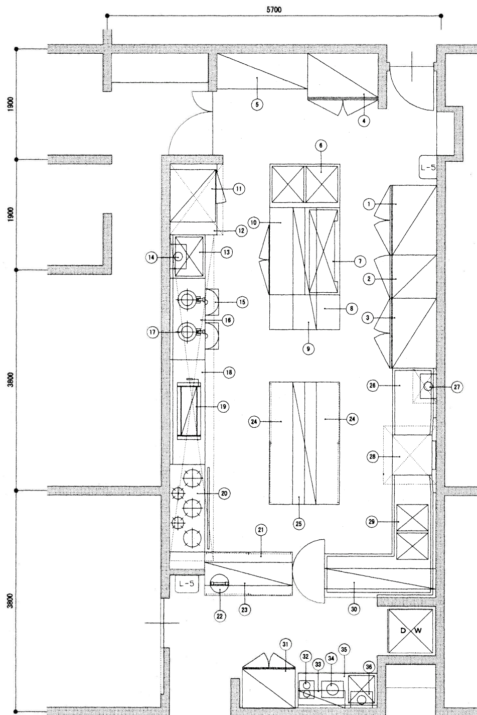
1 F 主厨房
